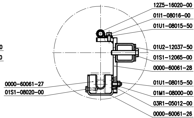
Schnitt C-C
