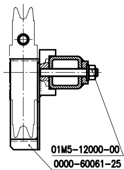
Schnitt A-A
